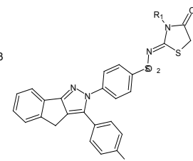
Scheme 19: R=C 6 H 5 , -CH 2 C 6 H 5 , -COC 6 H 5
