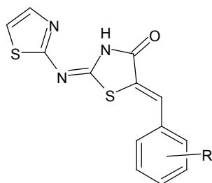
Scheme 2: R=H, 4-OH, OCH 3 , 3-OCH 3 , 4-OH, 2-NO 2 , 3-NO 2 , 4-NO 2 , 2-Cl, 3-Cl, 4-Cl
